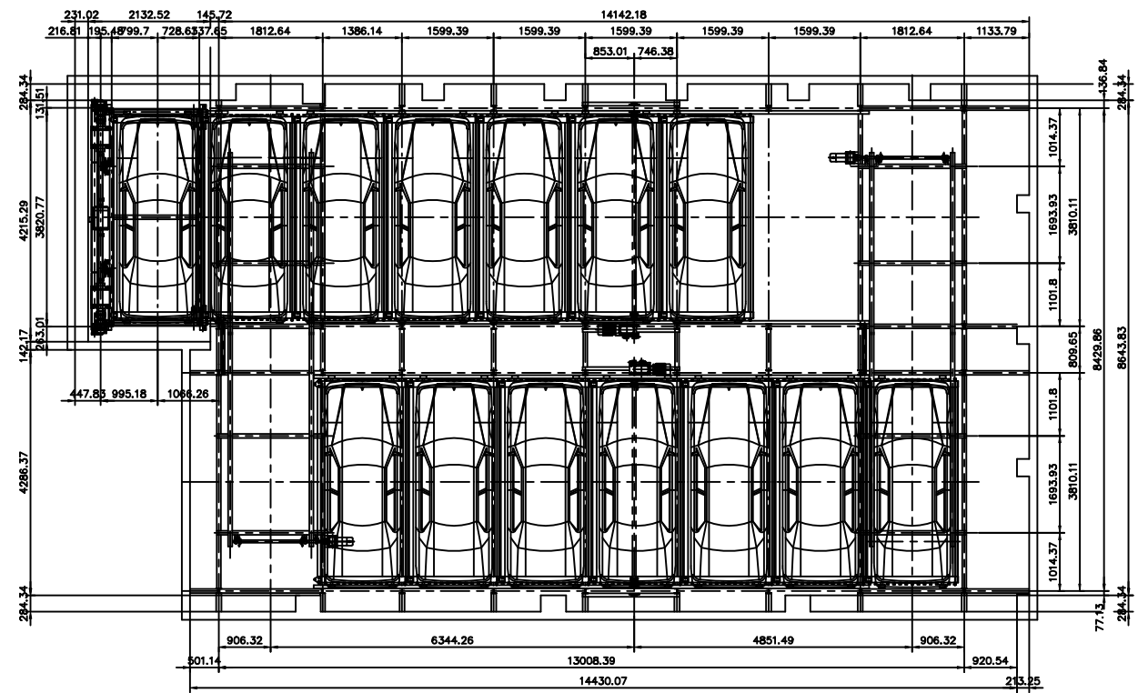
주차장 평면도 3 ( 지하 4층 )
