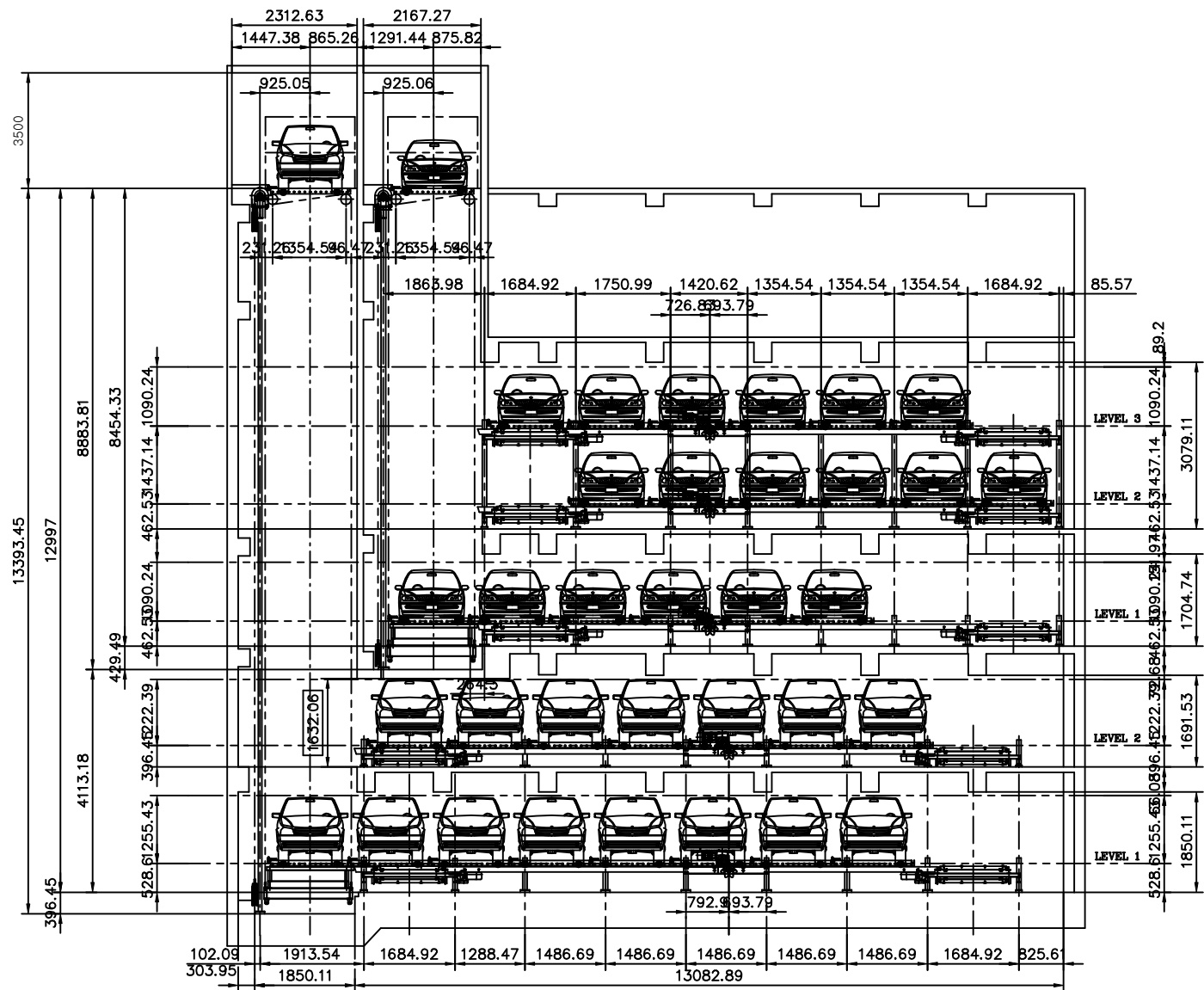
주차장 정면도
